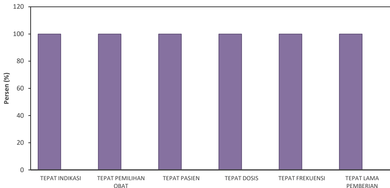
Gambar 2. Diagram Persentase Ketepatan Antipsikotik
